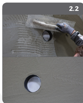
Udførelse af filslag for færdig gørelse af underpuds.
