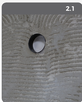
Udførelse af 1. lag underpuds med armeringsnet.
